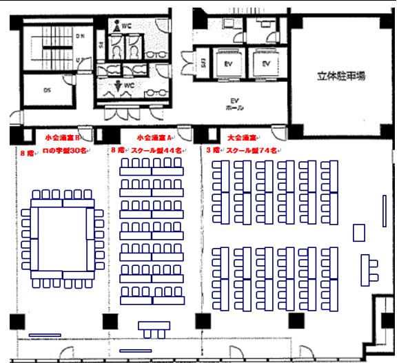
【3階・8階フロア図】
